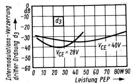
Bild 2. Intermodulationsverzerrungen dritter Ordnung ( d_3 ) als Funktion der Spitzenleistung (PEP) eines SSB-Transistors (40 V/50 W) mit der Speisespannung als Parameter
