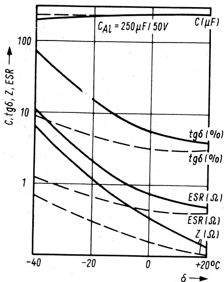
Bild 4. Temperaturverhalten eines Al-Elektrolyt-Kondensators 250\mu\text{F}/50\text{V} im Vergleich zwischen wasserhaltigem Glykol-Elektrolyten (Linie) zu einem organischen Elektrolyten (gestrichelt)
