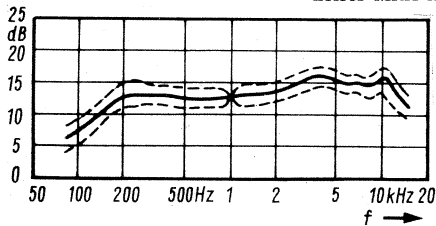
Bild 5. Frequenzkurve des Richtmikrofons MD 402 LM
