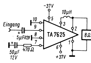
Bild 6. Äußere Beschaltung des Hybrid-Bausteines TA 7625 von RCA. Das Bauelement enthält einen kompletten 50-W-Nf-Verstärker
