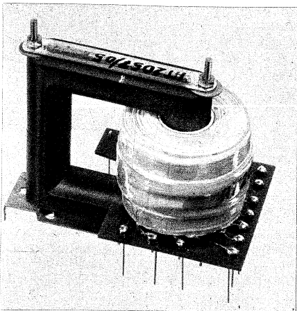
◀ Bild 7. Kombiniertes Horizontalablenk-/Hochspannungstransformator AT 2057/05 von Valvo für die 110^\circ -Eintransformatorenschaltung
