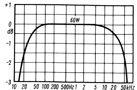
Bild 7. Frequenzgang der Schaltung nach Bild 6
