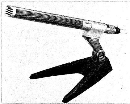
Bild 4. Rohr-Kondensator-Richtmikrofon Sennheiser MKH 415
