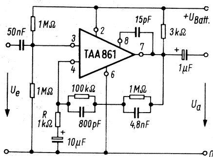
Bild 5. Die gleiche IS wie in Bild 4 wird in dieser Applikation als Entzerrungsverstärker für magnetische Tonabnehmer verwendet
