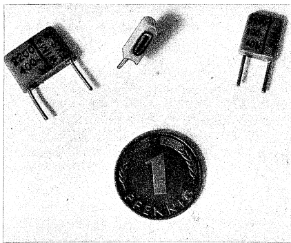
Bild 4. Kunststofffolienkondensatoren der Baureihen FKS 2 und FK 2. Zu beachten bei dem Schnitt in der Mitte ist die geringe Wandstärke. Der rechte Kondensator hat das Rastermaß 5 (Aufnahme: Schwahn)
