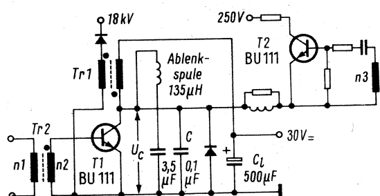
Bild 1. Vereinfachte Horizontal-Ablenkung nach dem Pump-Konzept
