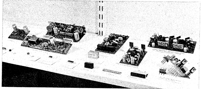
Bild 2b. ▼ Steckbare Bausteine des Scott-Receiver nach Bild 2a
