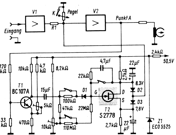
Regelautomatik eines Tonbandgerätes. Der fehlerhafte FET T2 schloß bei Aufnahme und Wiedergabe die Nf-Spannung kurz
