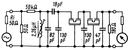
Bild 5. Meßschaltung des Fünfkreis-Hybrid-Keramikfilters der Stemag
