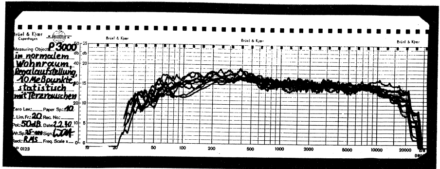
Bild 18. Original-Registrierstreifen einer Schalldruckmessung im normalen Wohnraum mit einem Lautsprecher P 3000
