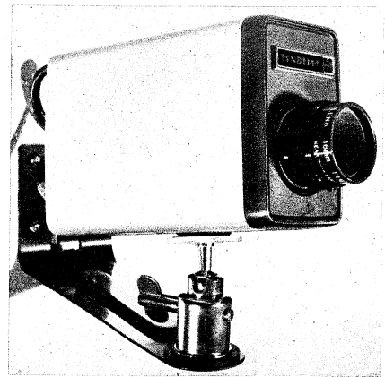
Bild 4. Sehr einfach aufgebaute Überwachungskamera von Matsushita. Die Schärfereinstellung erfolgt mit Hilfe des Objektivs (Aufnahme: Schwahn)
